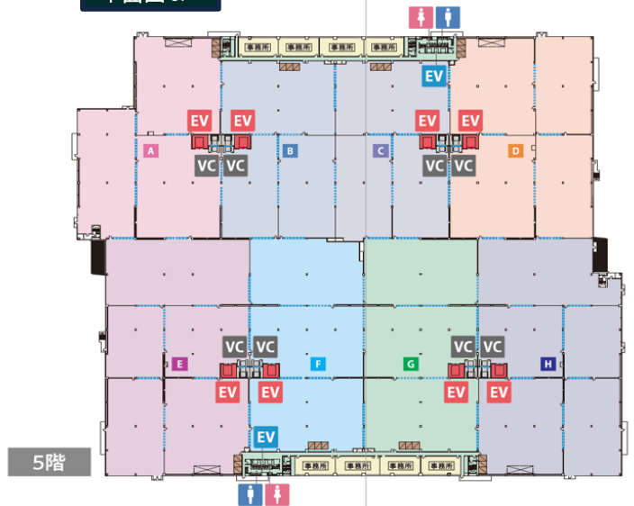
平面図 5F
