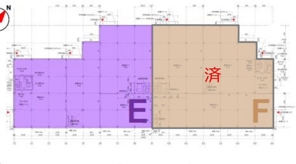
2階 平面図
