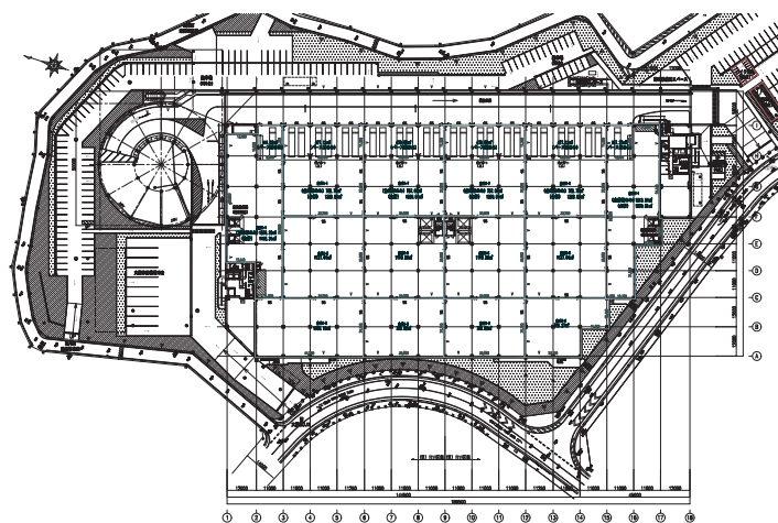
平面図 1F
