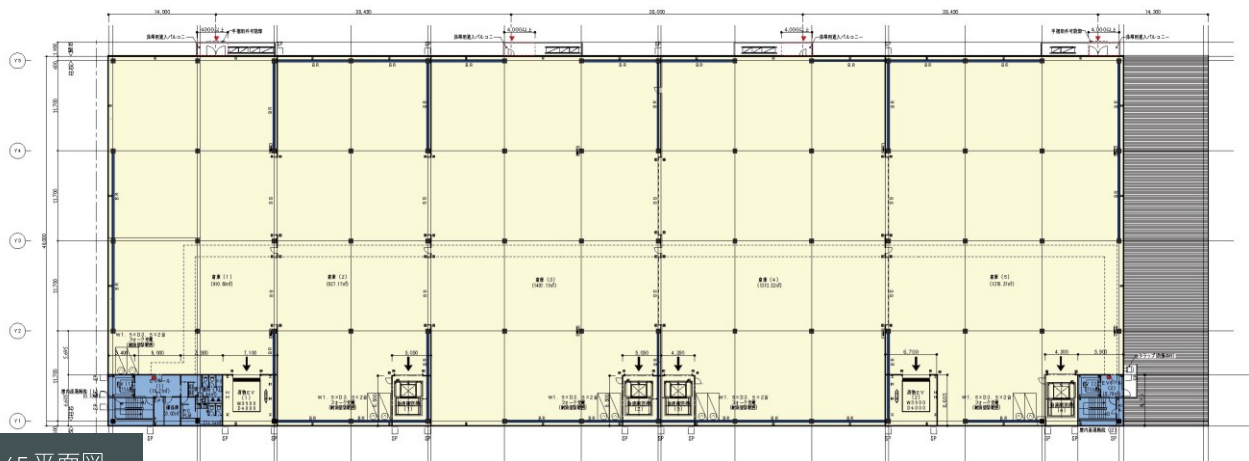
4F平面図
