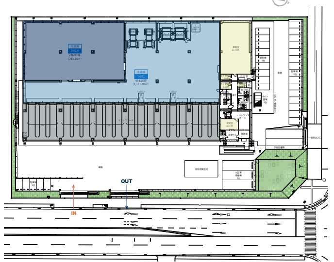
配置図・1F 平面図
