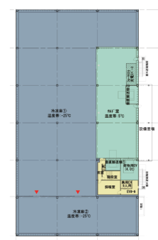
3-5F 平面図
