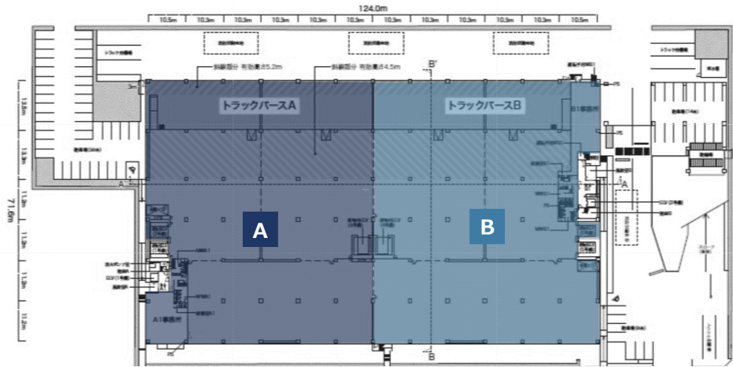
配置図・1階
